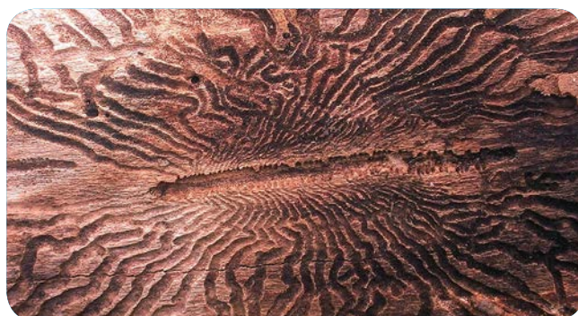
Domages causés par l'agrile du frêne
